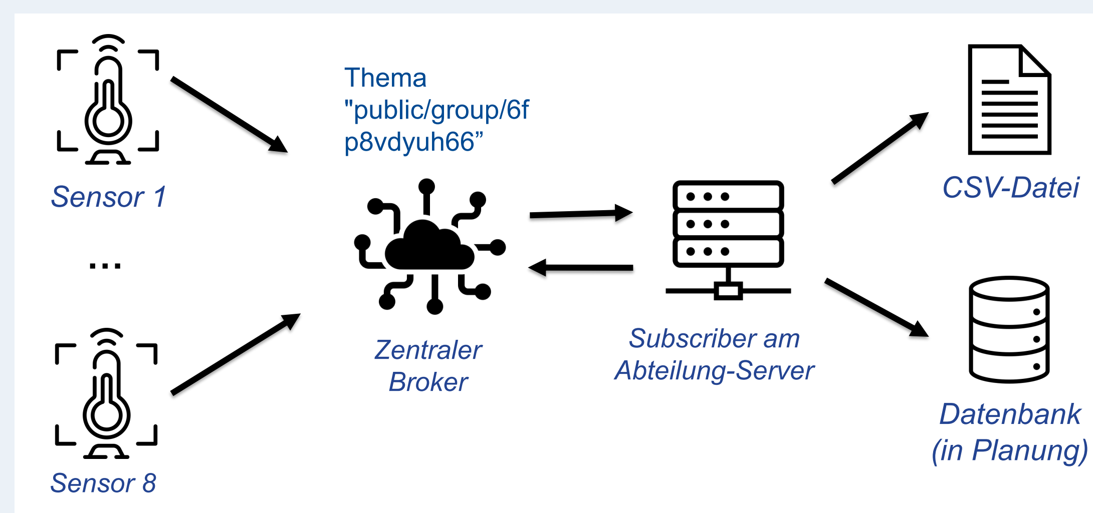
Abbildung 3. Arbeitsablauf der Datenerhebung und -speicherung
