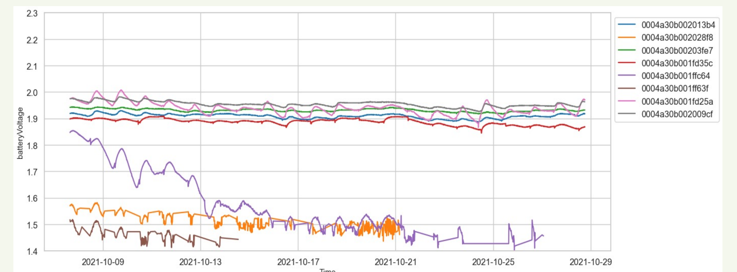
Abbildung 6. Batteriespannung nach Sensor-ID im Oktober 2021
