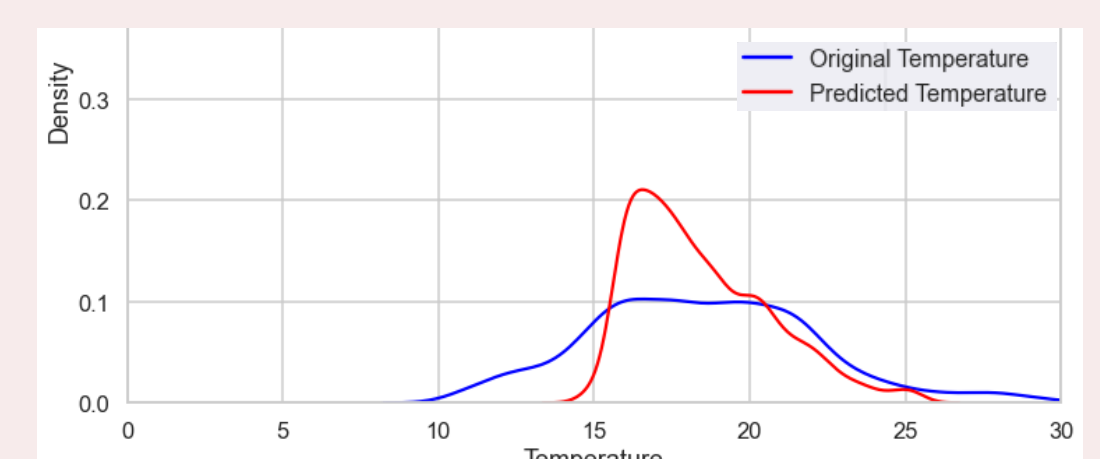
Abbildung 5. Verteilungsdiagramme der tatsächlichen und vorhergesagten Temperatur mit linearer Regression auf der Grundlage der Luftfeuchtigkeit im September 2021
