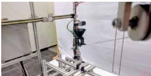
SEGESTA-Prüfstand mit drehbar gelagerten Umlenkrollen und beweglichen Basispunkten
